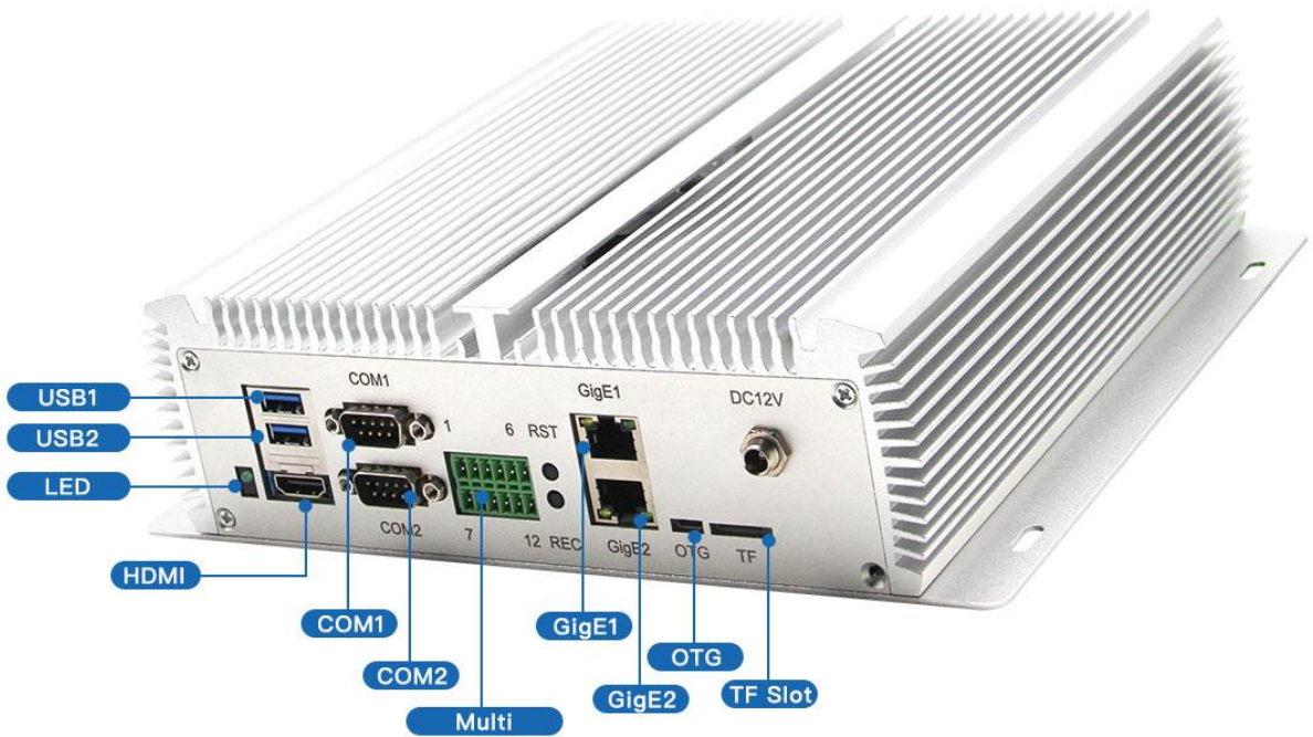
8F5E2 正面接口标识图
